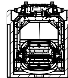
SCHNITT B-B
